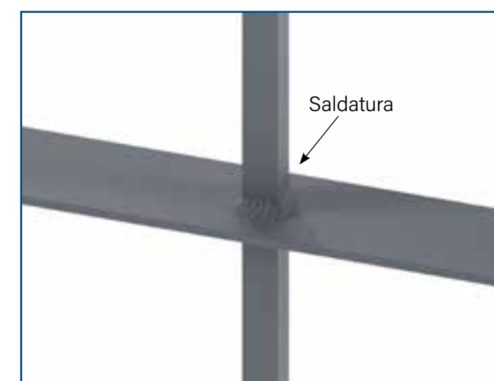
K QUADRO 14x14 mm + PIATTO
